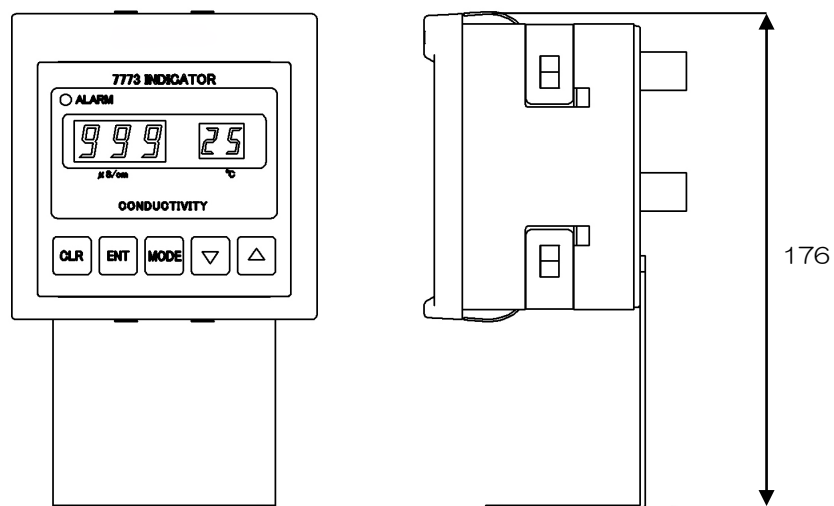
取付金具付き本体外形図
