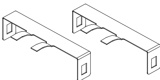
パネルマウント用金具 (付属) (7721-M100)
