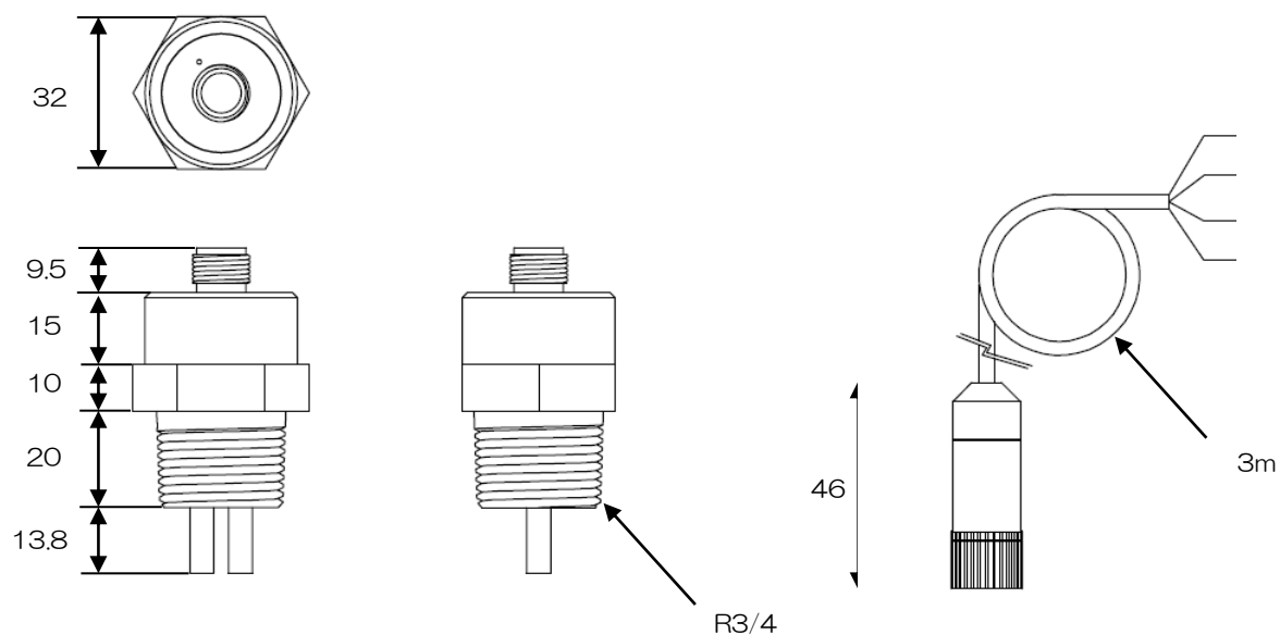
7770-S200 センサー外形図
