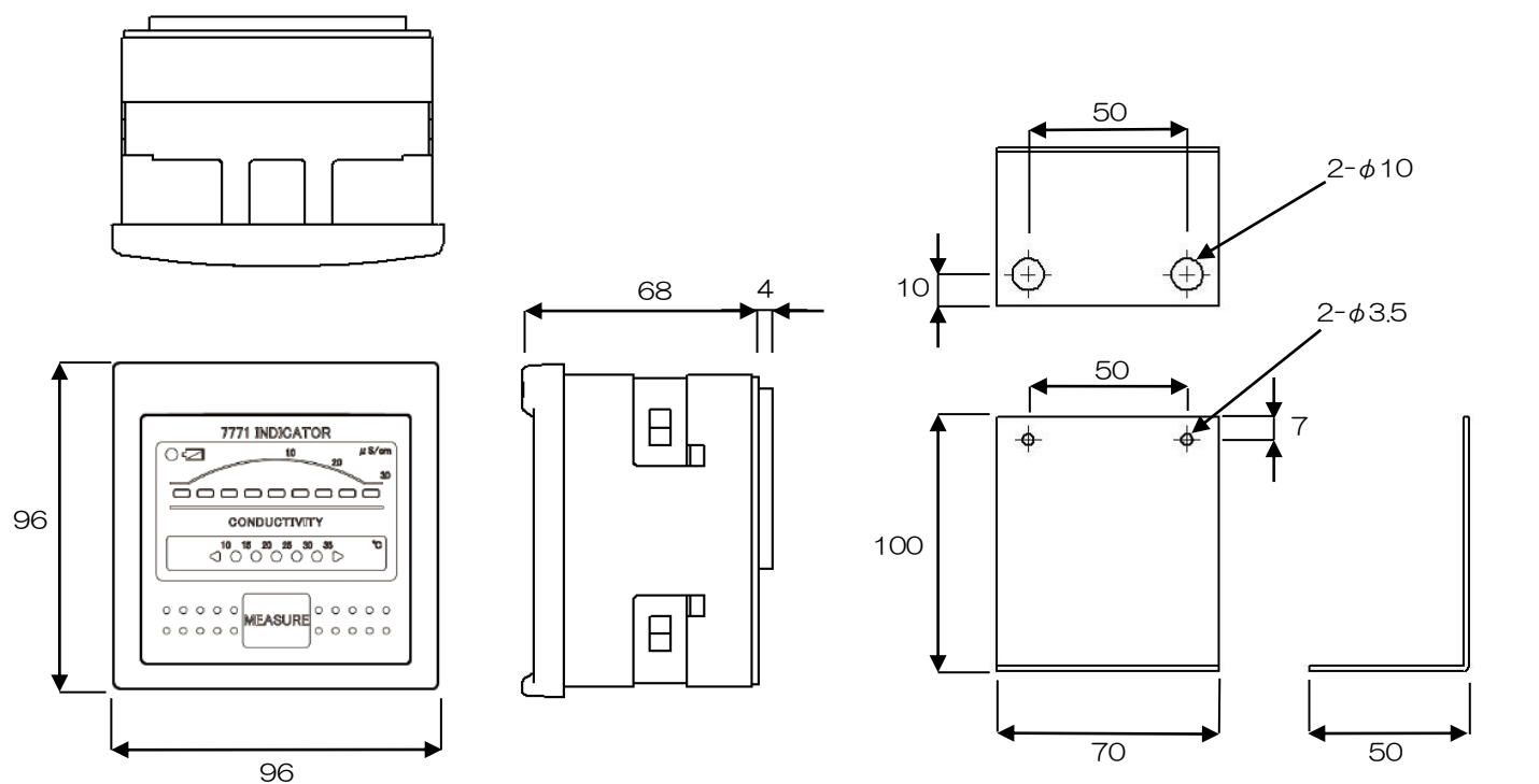
本体外形図
