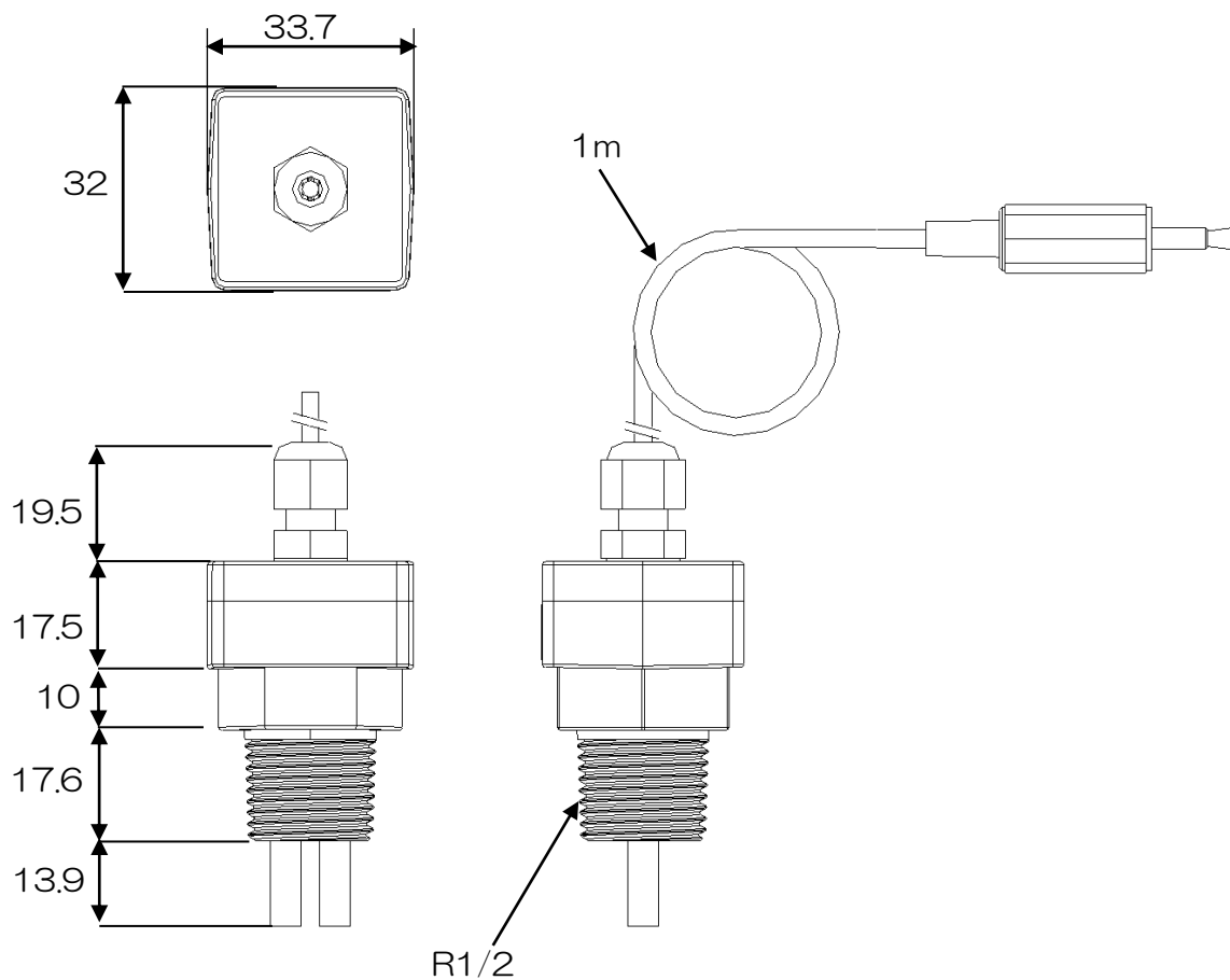
センサー外形図
