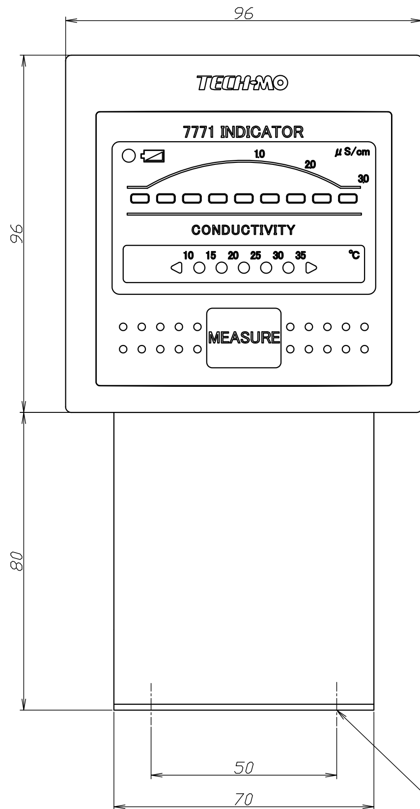
前面図
