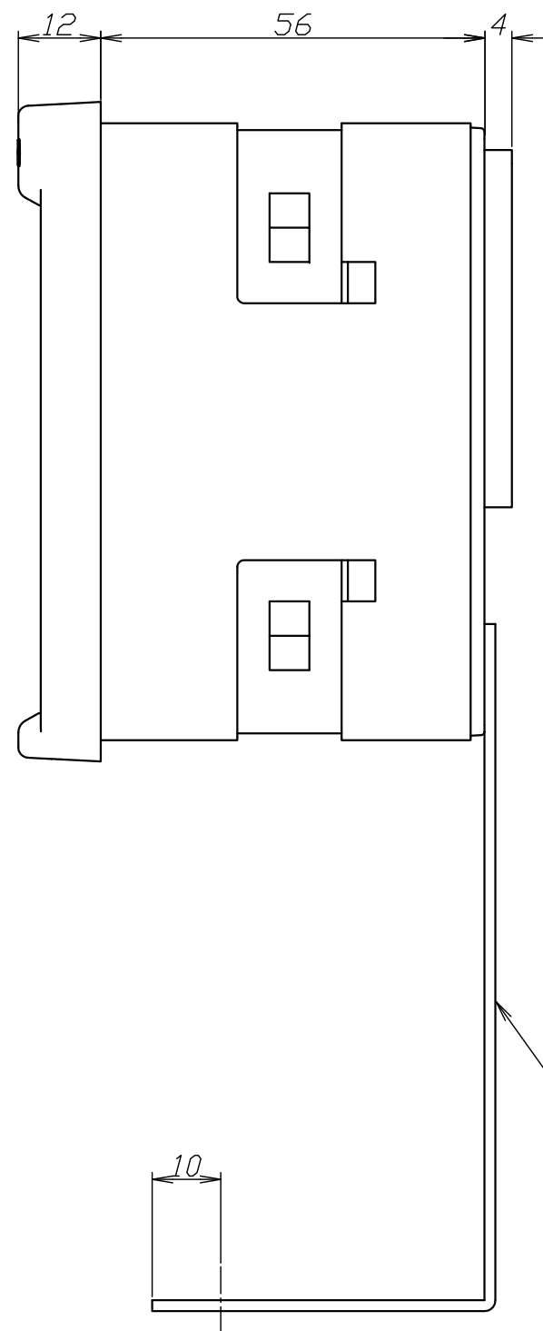
側面図
