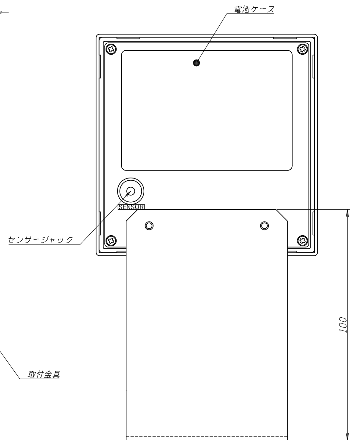
後面図
