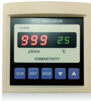
正面
