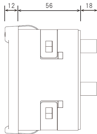
右側面
